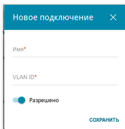
Рисунок 44. Добавление подключения.
